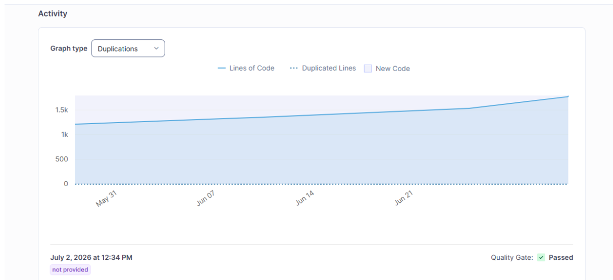
Figura 28: SonarQube Report - Indice di duplicazione
